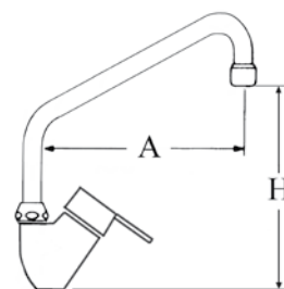
Medidas A 250 / H 215 mm (GF.97) A 300 / H 240 mm (GF.98)
